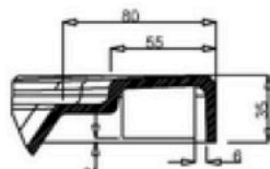
D SCALE 1:2
